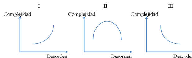
Ilustración 2. Las tres categorías de la complejidad como función del desorden. Figura extraída de Shiner, Davison y Landsberg (1999).
