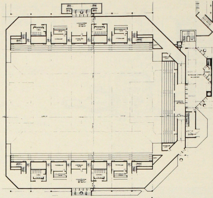
PLANTA DE INGRESOS 2º NIVEL
