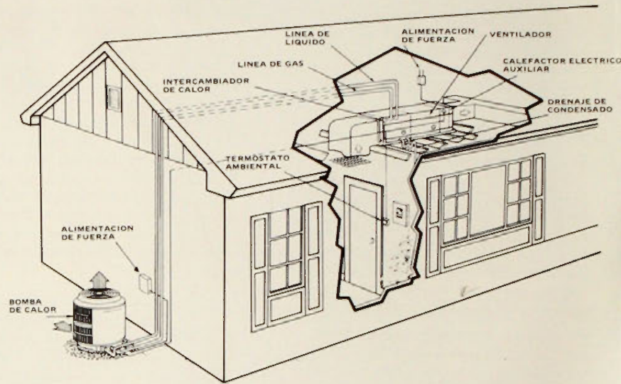
INSTALACION TIPICA DE BOMBA DE CALOR
