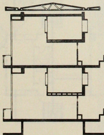
CORTE
