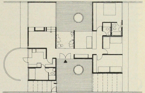
PLANTA
