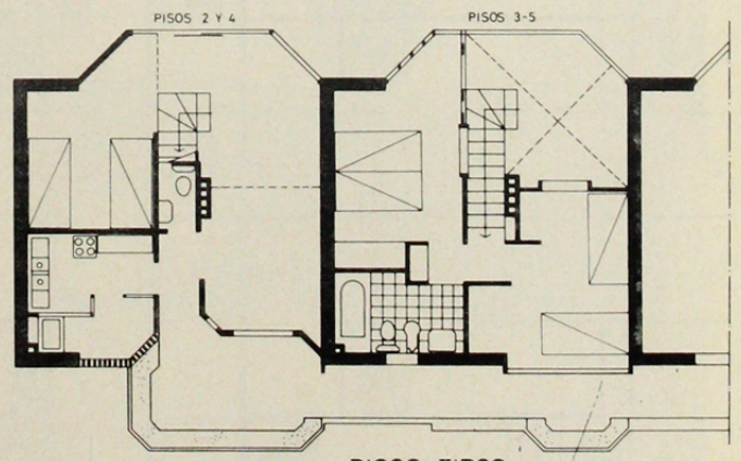
PISOS TIPOS
