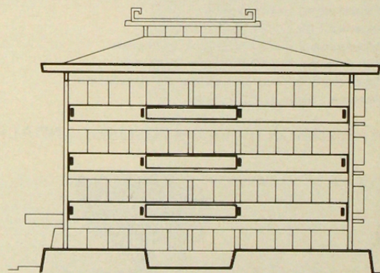
ELEVACION
