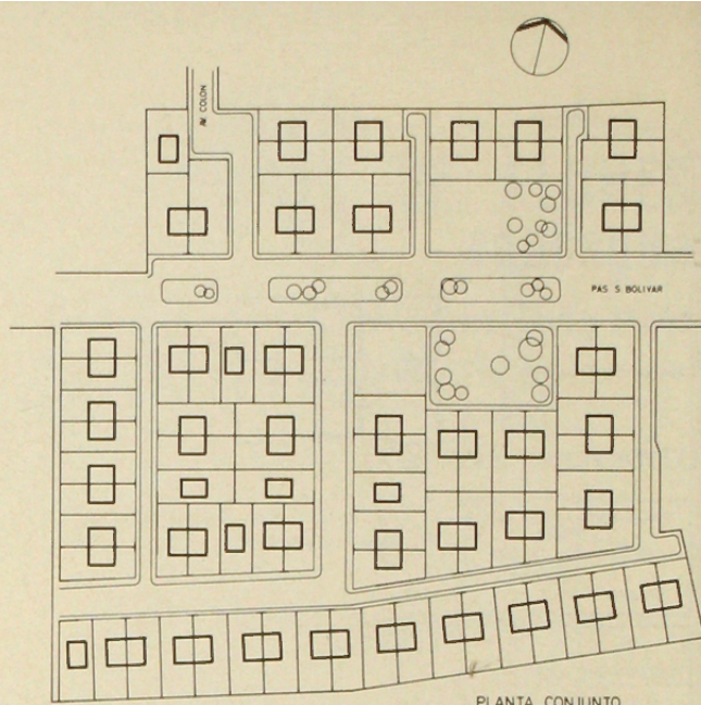
PLANTA CONJUNTO
