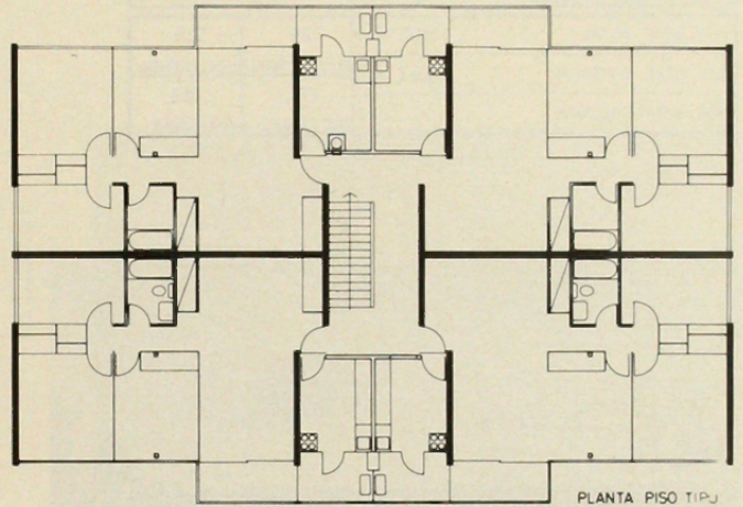
PLANTA PISO TIPO
