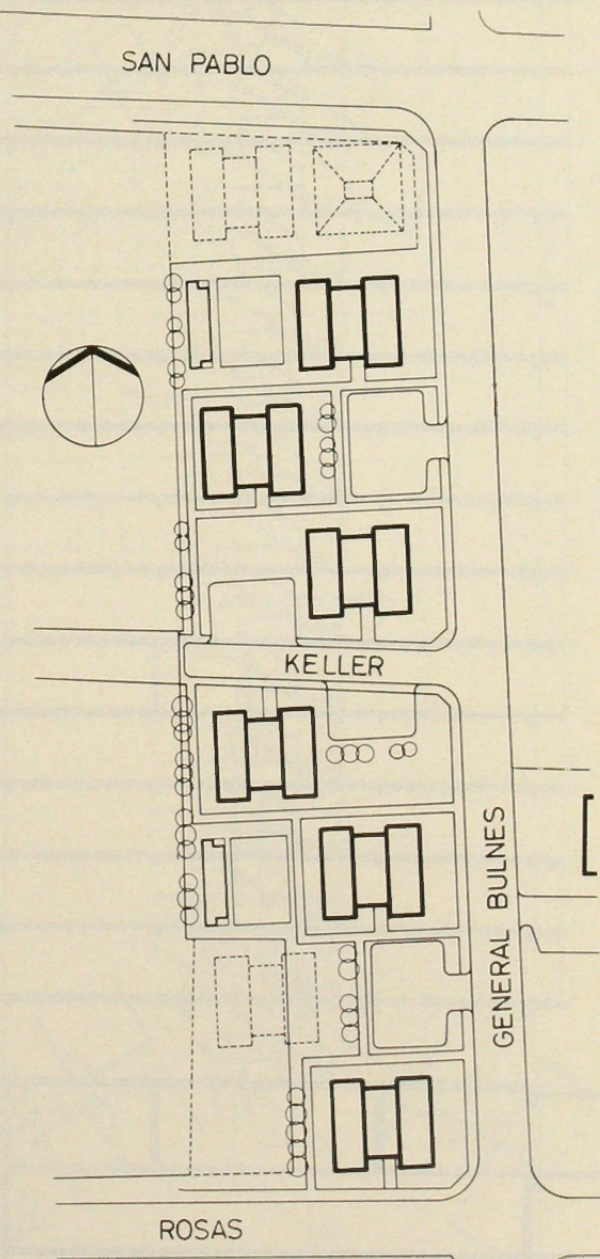
PLANO CONJUNTO
