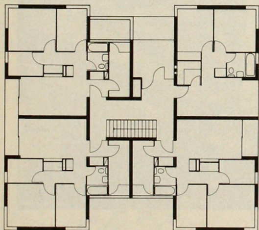
PLANTA 1er P
