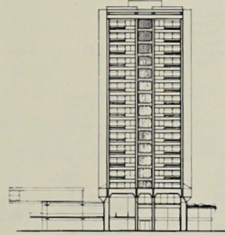
ELEVACION TORRE 2
