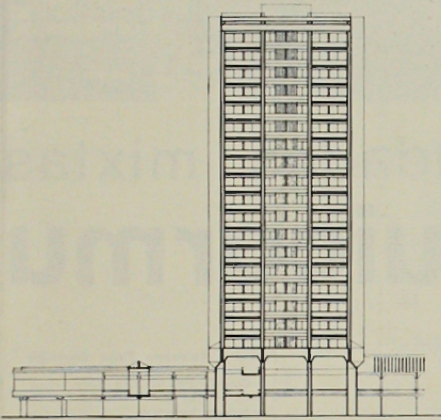
ELEVACION TORRE 1
