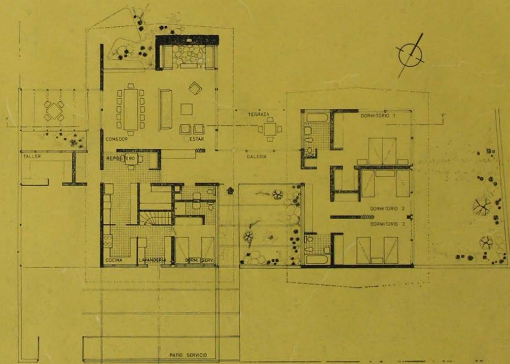
PLANTA
