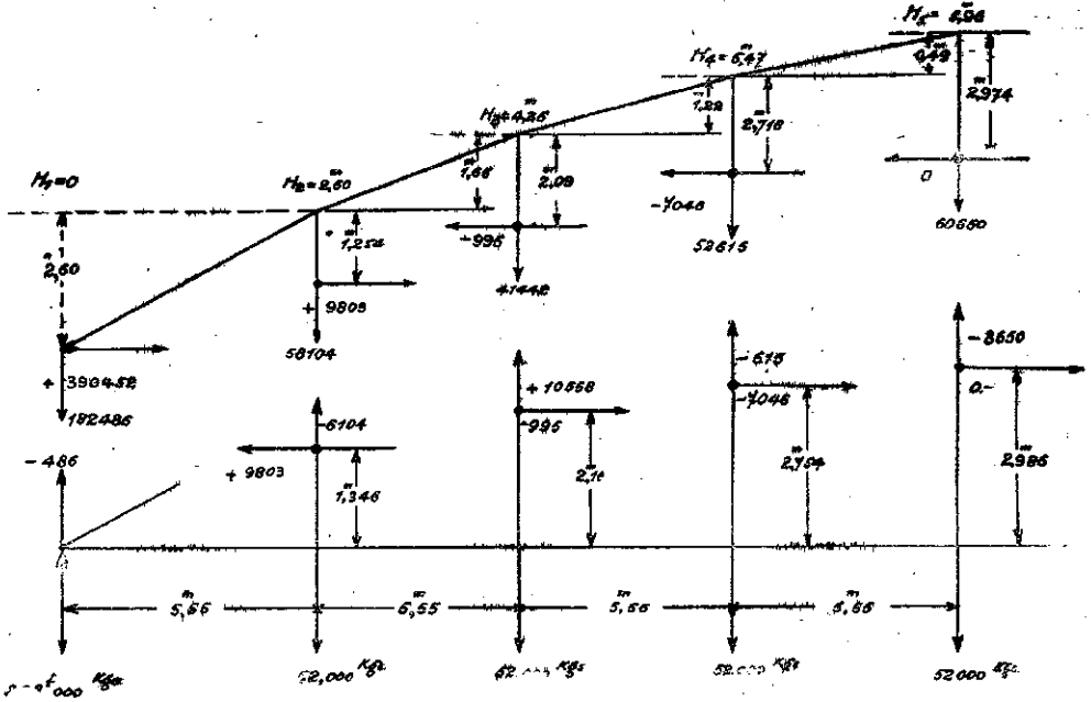
Momentos de las cargas horizontales \pi
